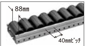
JB-590 静電 (40ピッチタイプ)
