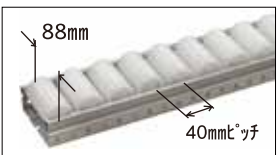
JB-590 (40ピッチタイプ)
