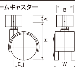
樹脂フレームキャスター
