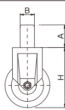
金属フレームキャスター 差し込み式 固定タイプ
